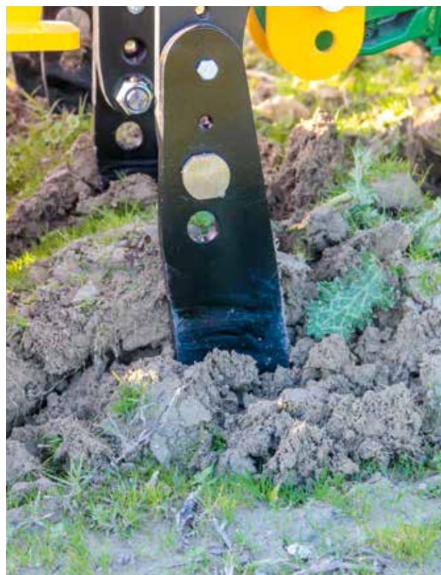
L'ameublisseur Combivigne peut travailler dans des vignes ayant un écartement inter-rang de 1,20 à 2,20 mètres. Il est ici associé à une herse rotative Agrisem.
